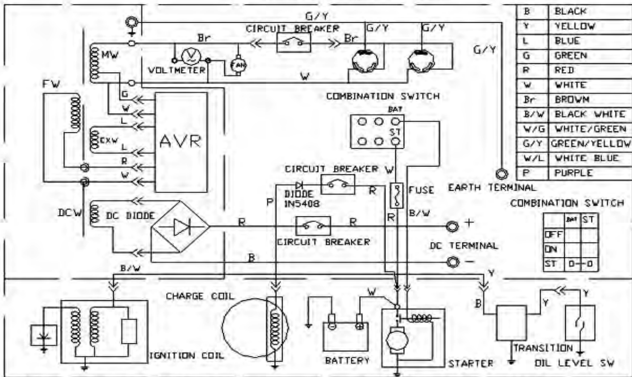
CC5000-G-B 220V/50Hz 燃气发电机组电路图
